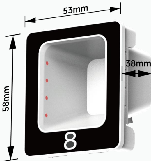
外壳尺寸
