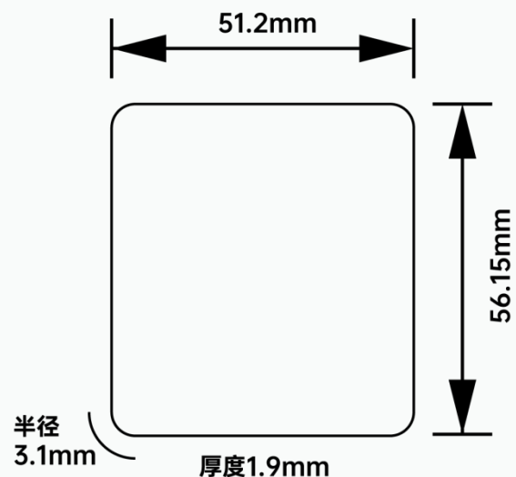
不锈钢开孔尺寸
